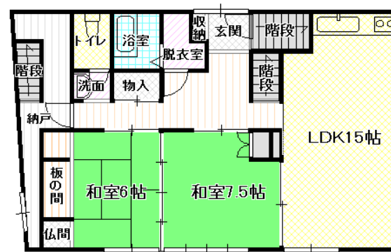
2階現況優先
