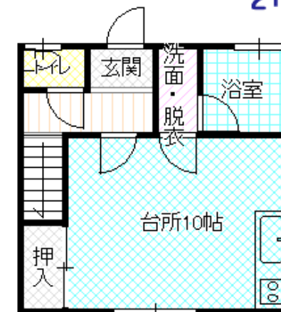
1F 現況優先
